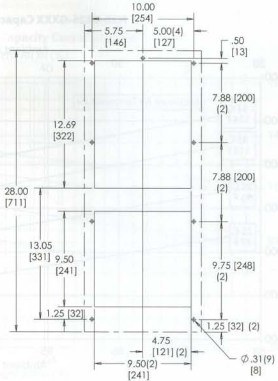
Cutout Dimensions
