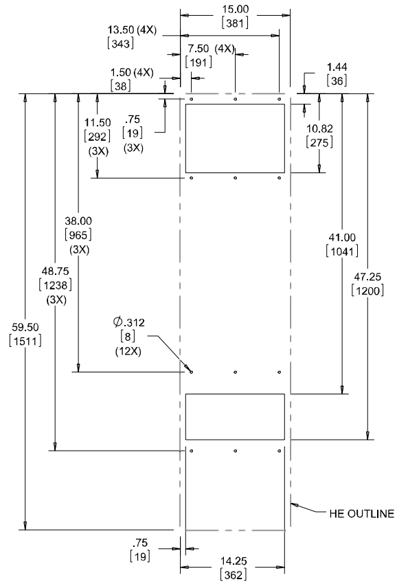
Cutout Dimensions
