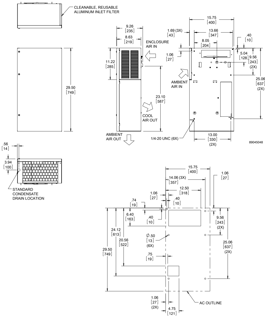
Cutout Dimensions
